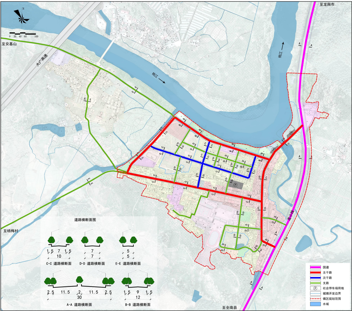
镇区道路交通规划图
