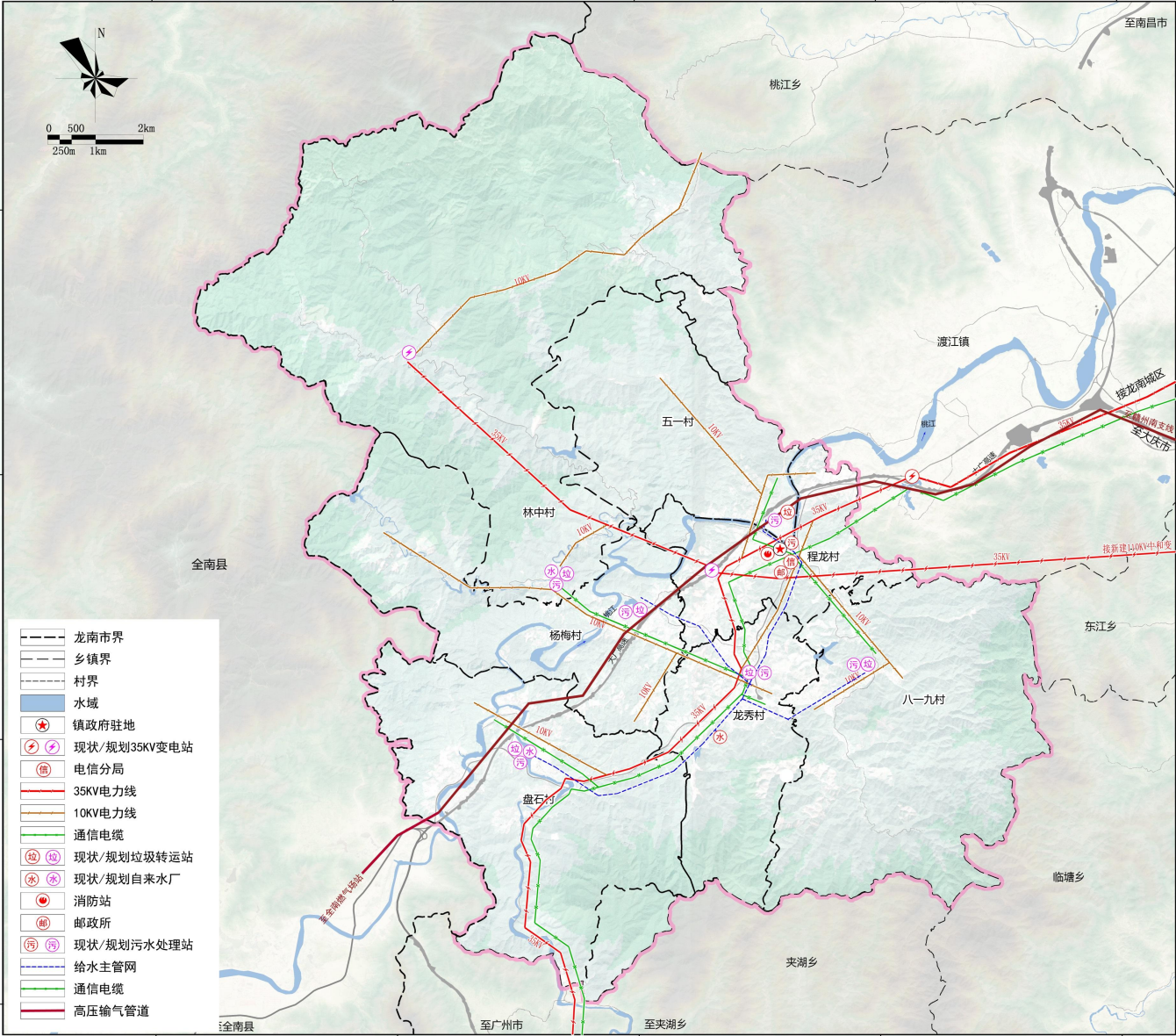
镇域基础设施规划图
